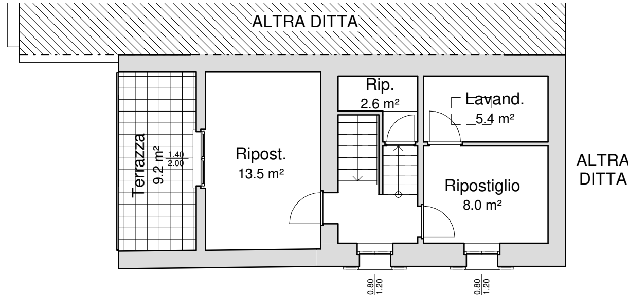
PIANO SECONDO
