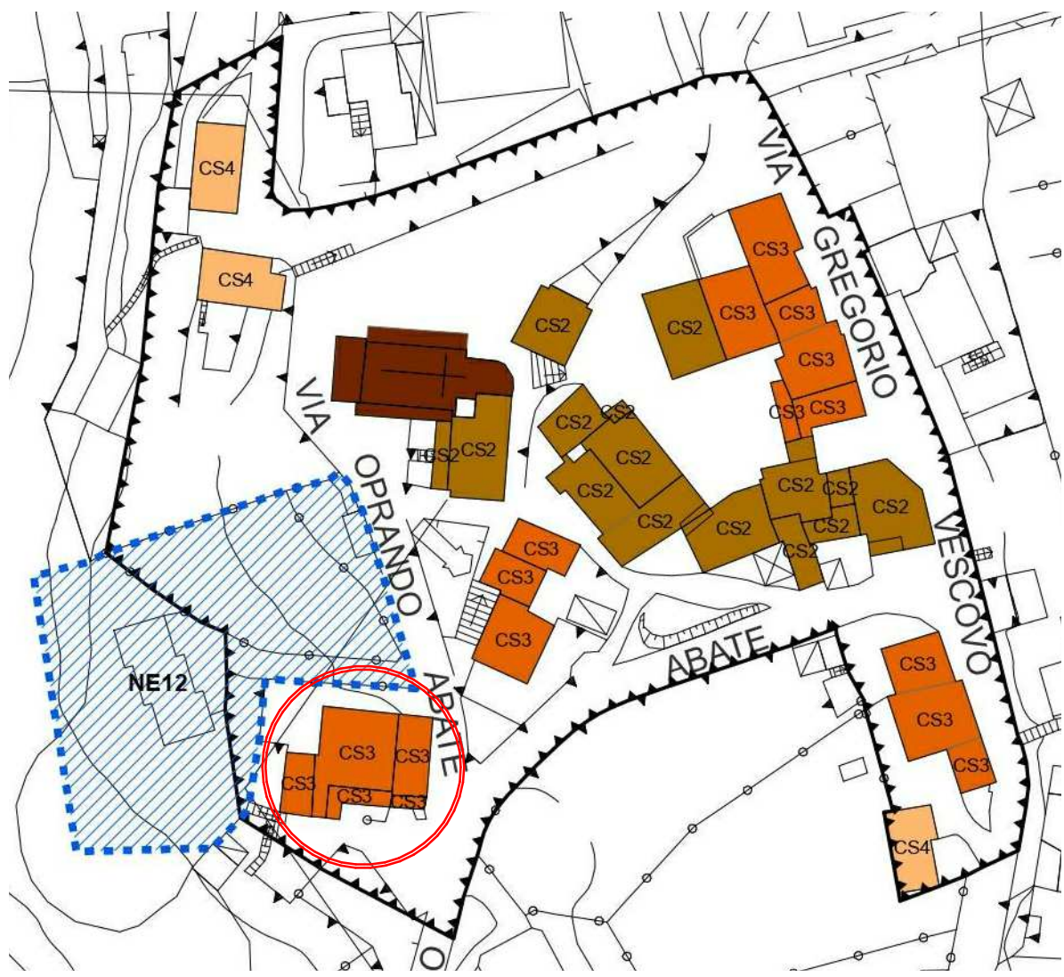
ESTRATTO PGT 1 : 1000
