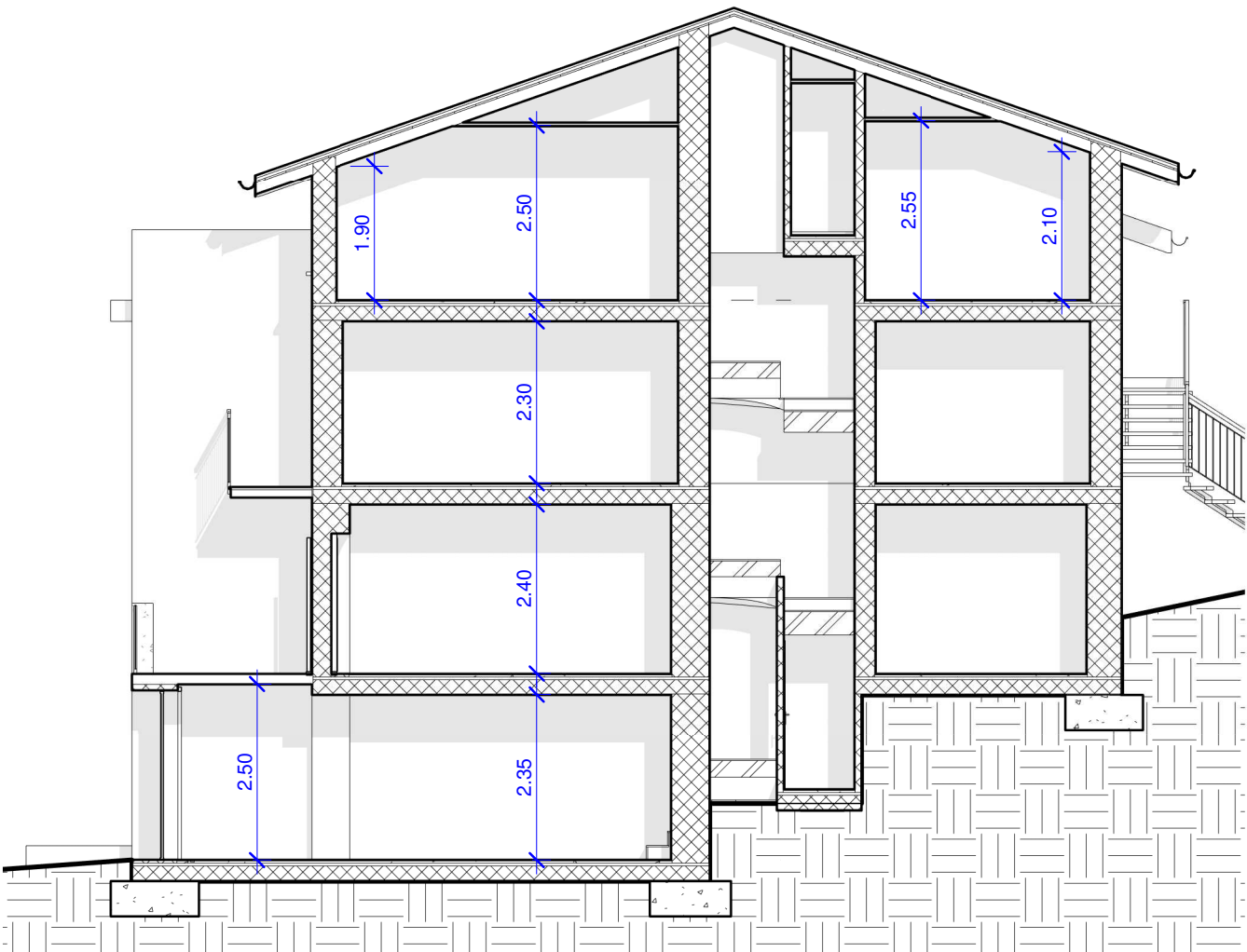
SEZIONE A-A
