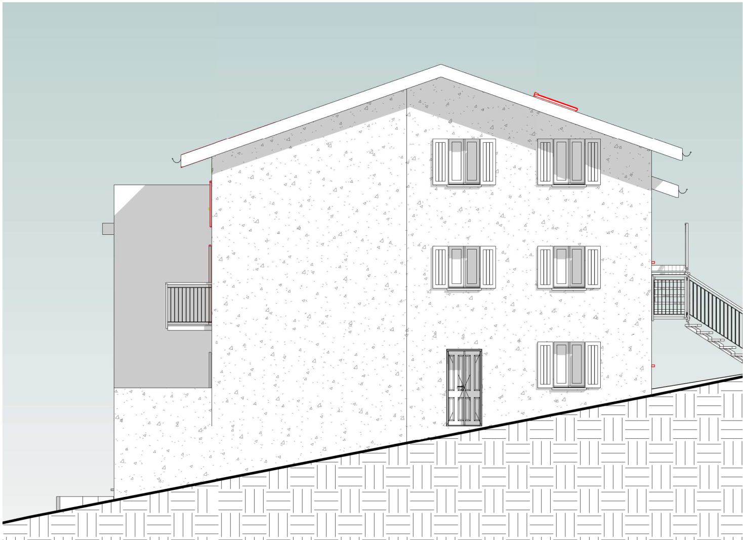
PROSPETTO EST
