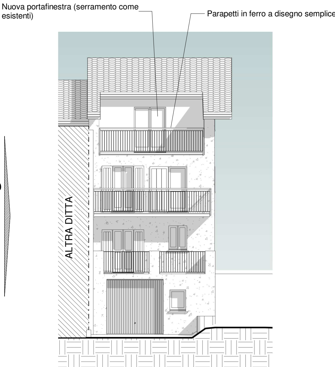
PROSPETTO SUD
