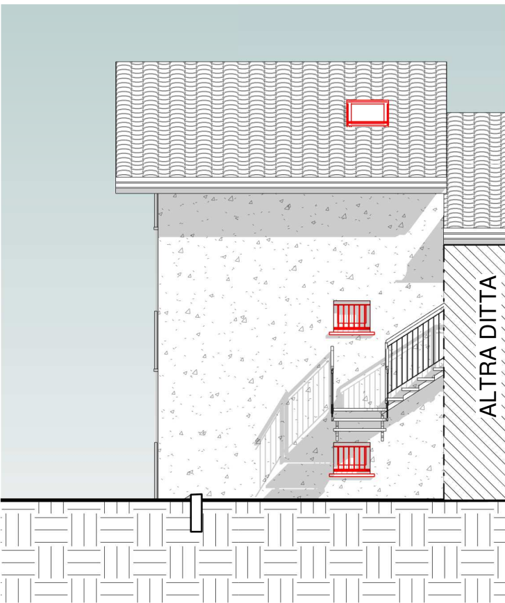
PROSPETTO NORD
