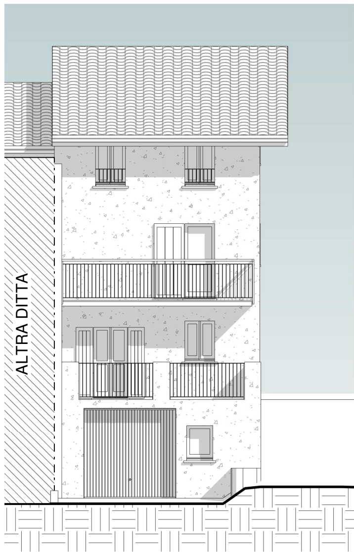
PROSPETTO SUD
