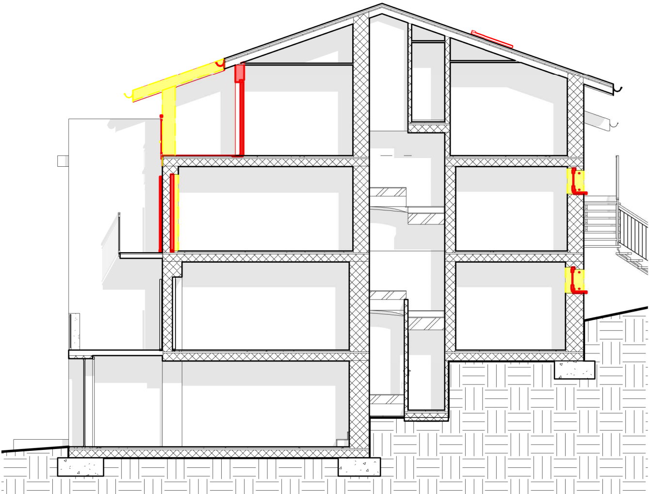
SEZIONE A-A
