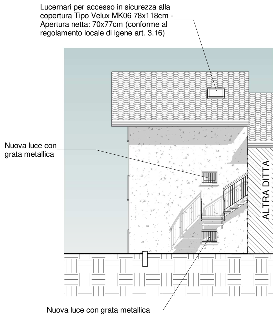
PROSPETTO NORD
