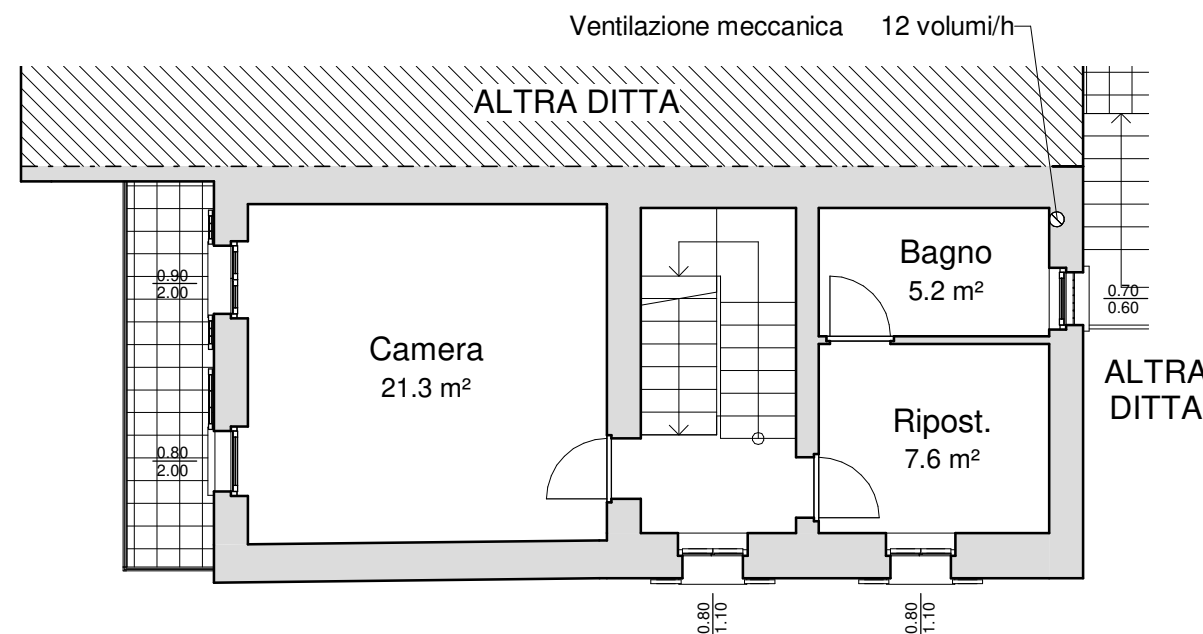
PIANO PRIMO
