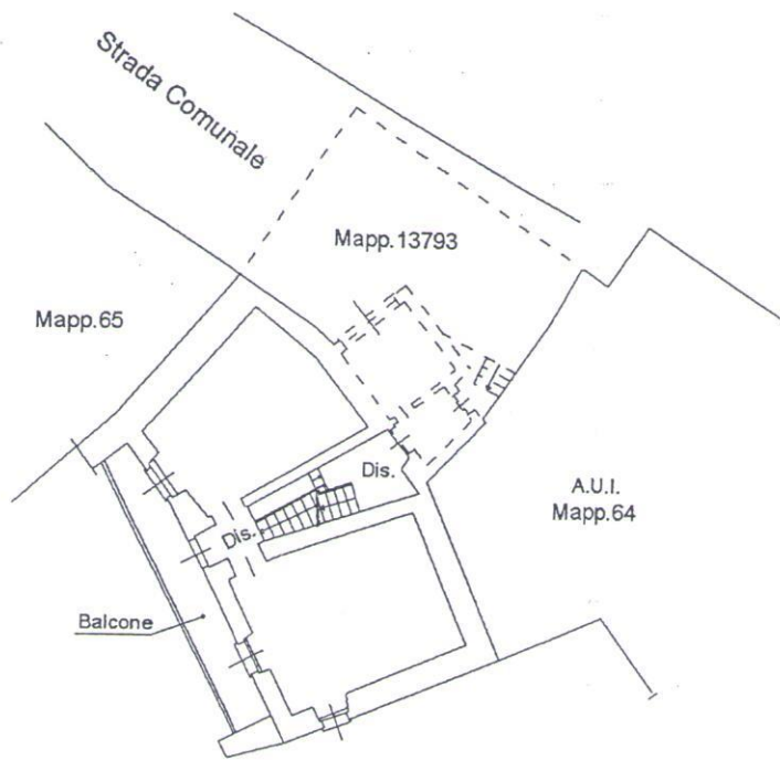
PIANTA PIANO PRIMO H=mt.2.70
